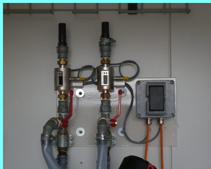
Débitmètre électronique
