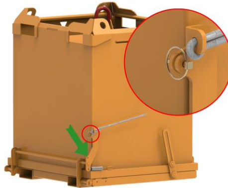
Levier verrouillable
