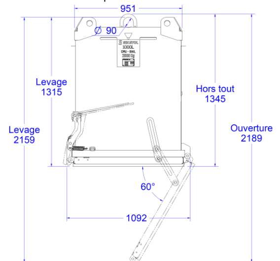
Passages de fourches en parties supérieure et inférieure
